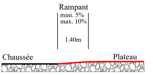
Coupe de principe sur plateau traversant
