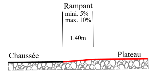
Coupe de principe sur plateau traversant
